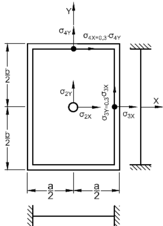
FIG.7 ALL EDGE RIGIDLY FIXED
