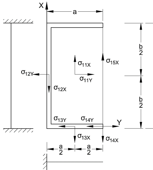
FIG. 10 THREE EDGES FIXED AND ONE LONG EDGE FREE
