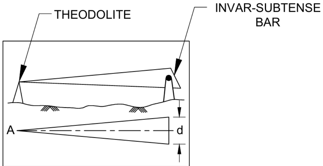
FIG. 4 USE OF INVAR-SUBTENSE BAR
