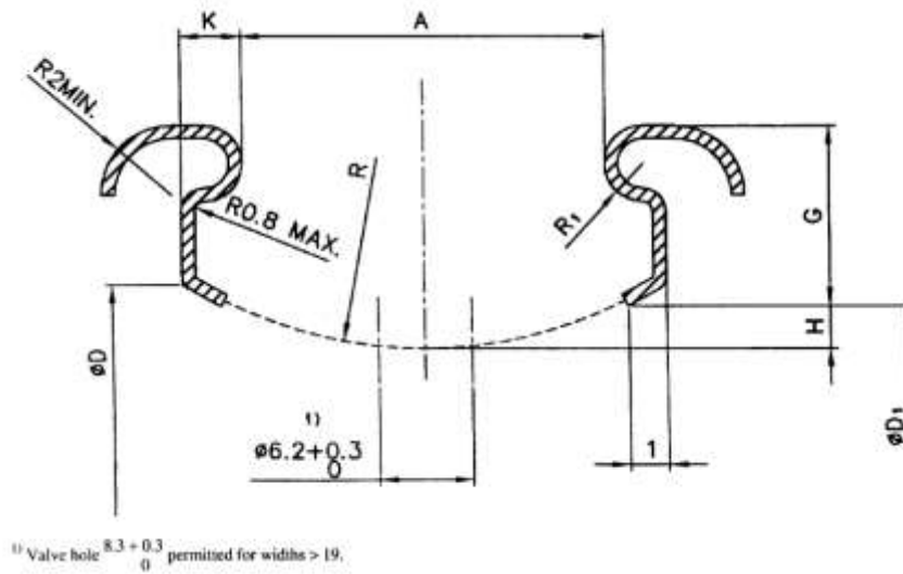
FIG. 5 CROCHET RIMS
