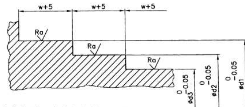
FIG. 27 TAPE MANDREL
