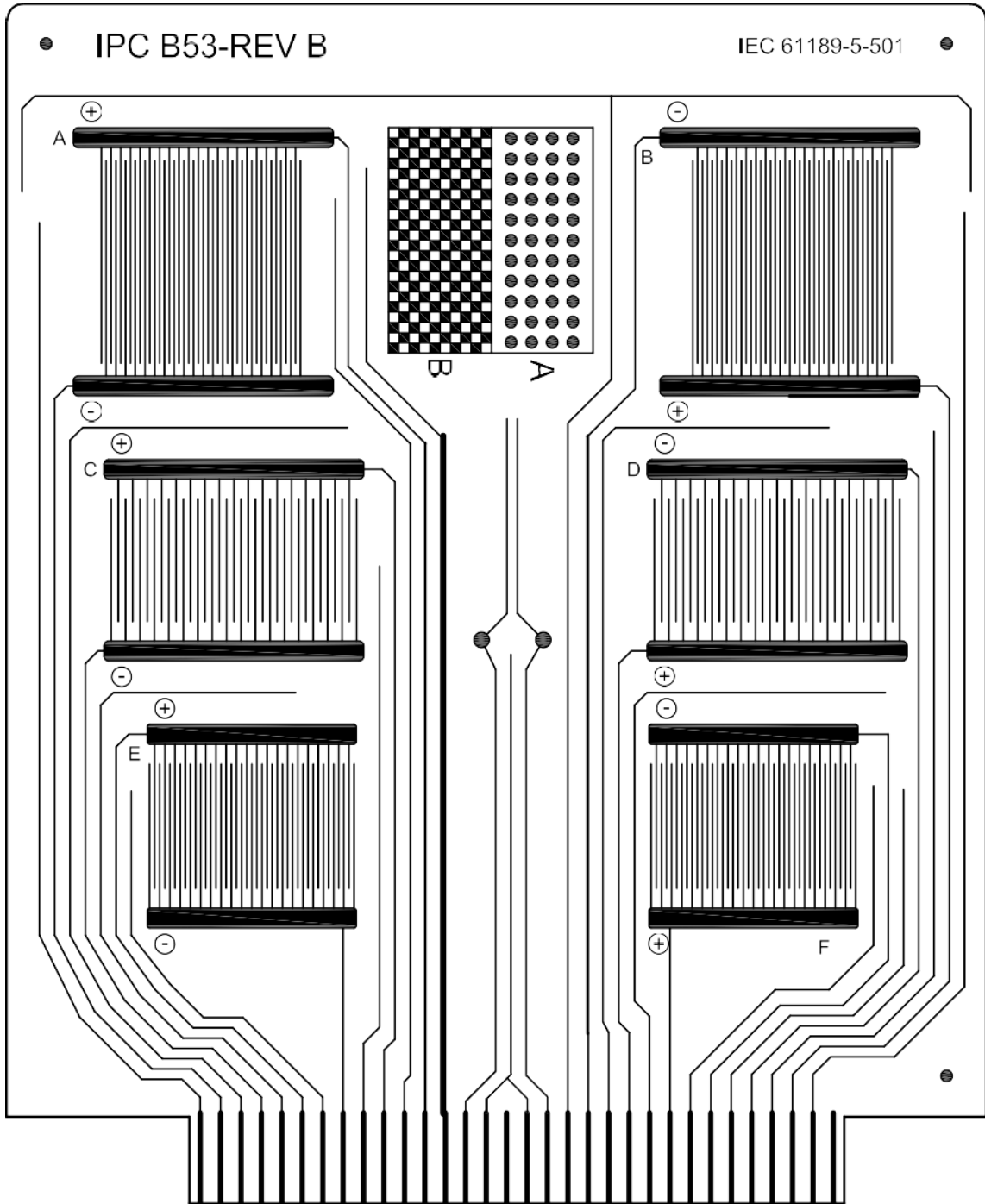
FIG. 10 IPC B53-REV B TEST COUPON (SOURCE ISO 9455-17 : 2024)
