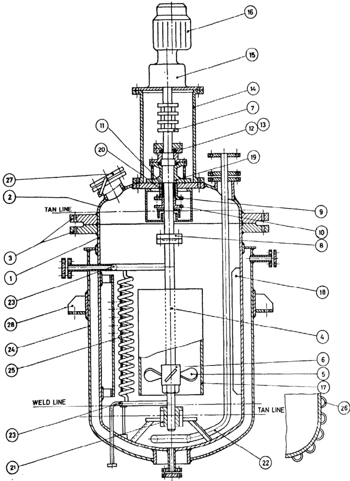
FIG. 1 AGITATOR ASSEMBLY
