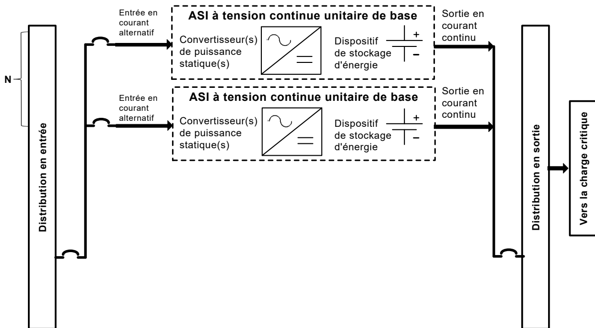
Figure A.2 – Système dimensionné pour la charge ( N unités d'ASI à tension continue) – Sans redondance
