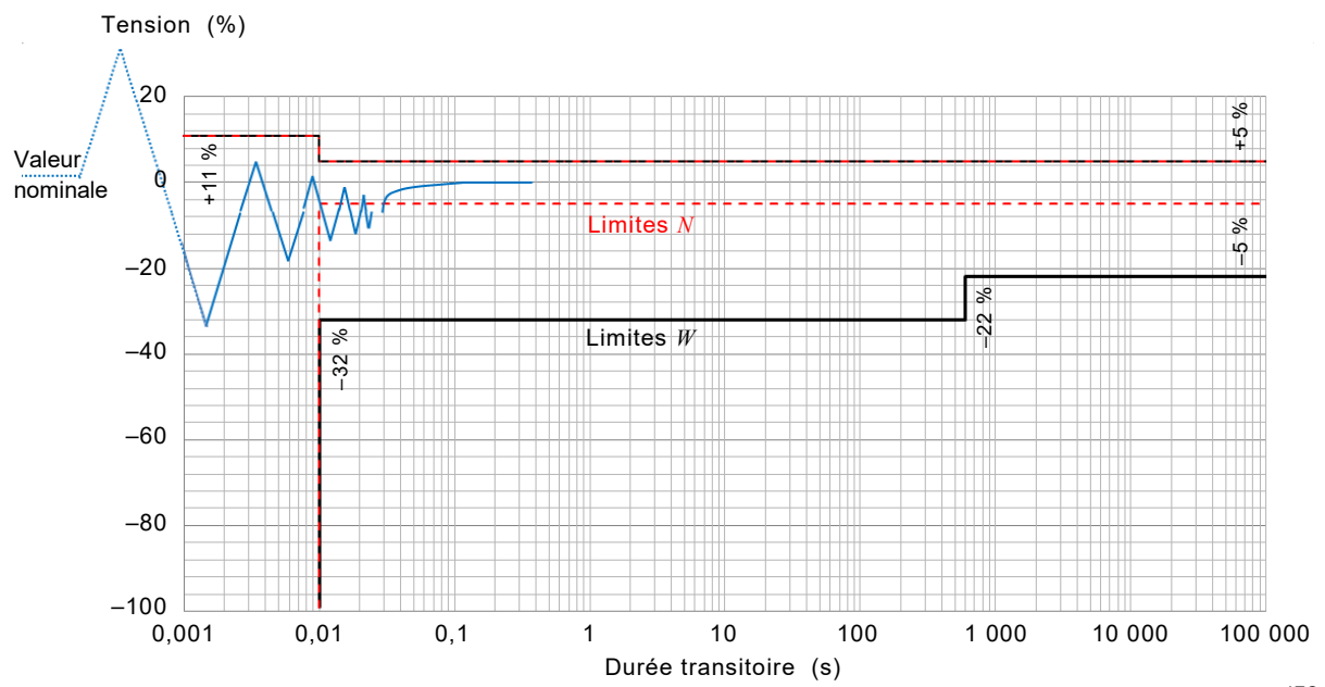
Figure E.2 – Exemple: Validation de la réponse en tension dynamique avec la limite large bande
