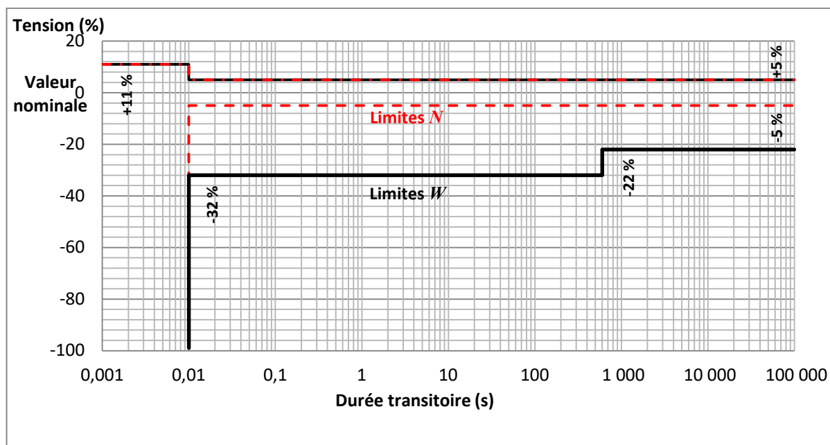
Figure 2 – Performances dynamiques de sortie
