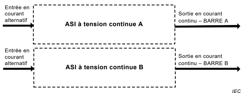
Figure A.5 – ASI à tension continue à double voie de distribution
