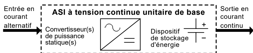
Figure A.1 – ASI à tension continue unitaire de base
