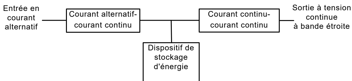
Figure B.2 – Topologie à convertisseur série
