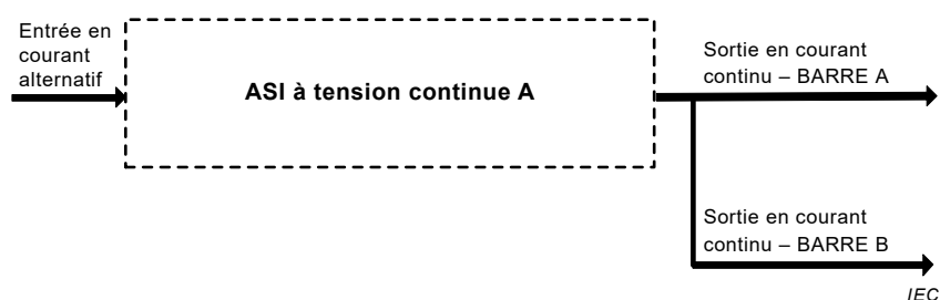
Figure A.6 – Variante d'ASI à tension continue à double voie de distribution
