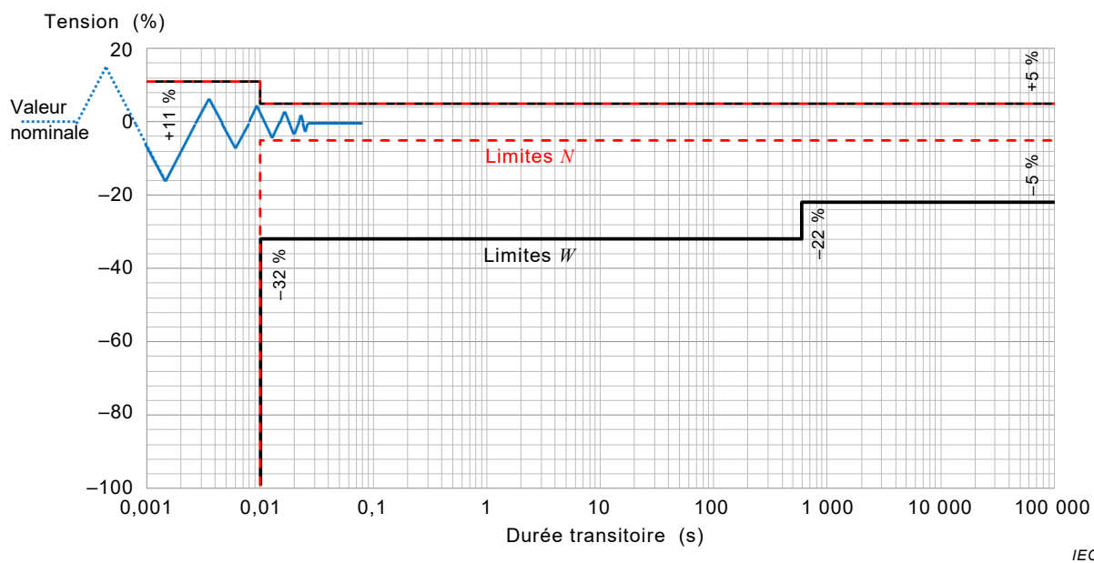
Figure E.1 – Exemple: Validation de la réponse en tension dynamique avec la limite bande étroite
