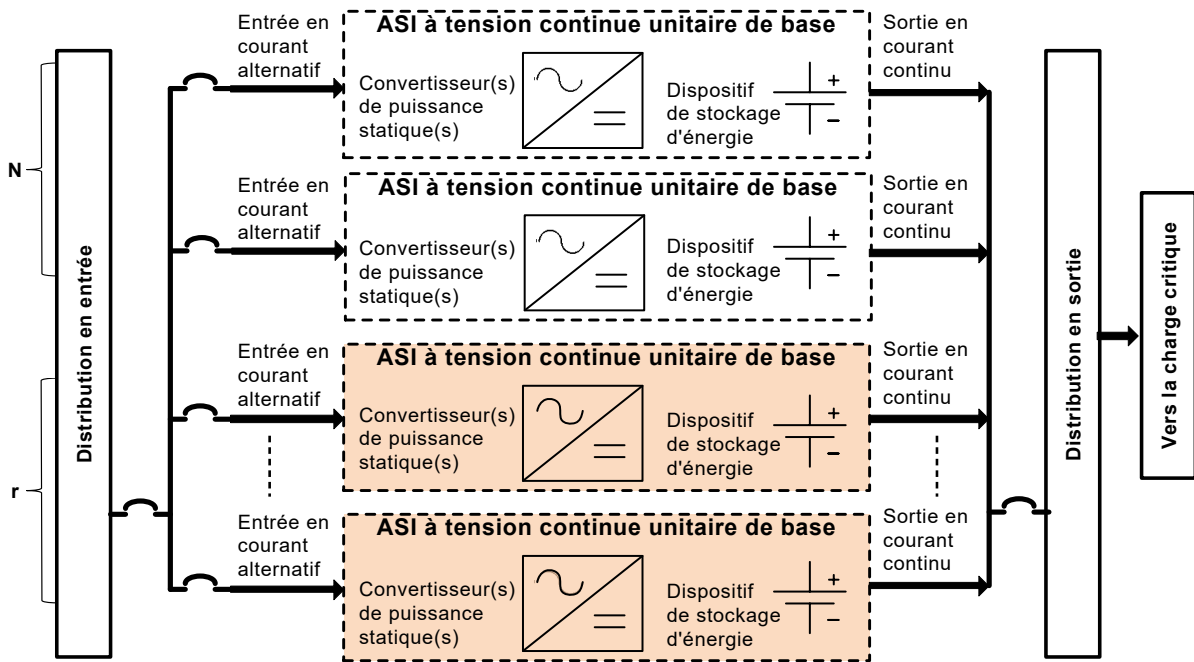
Figure A.4 – Système dimensionné pour la charge ( N unités d'ASI à tension continue) – Redondance N + r
