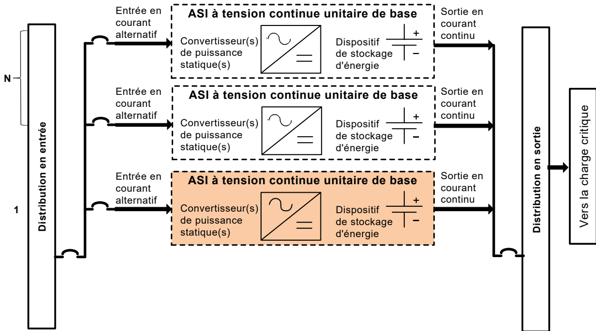
Figure A.3 – Système dimensionné pour la charge ( N unités d'ASI à tension continue) – Redondance N + 1
