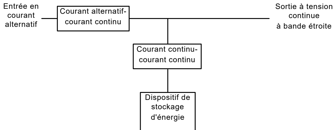
Figure B.3 – Topologie à convertisseur parallèle
