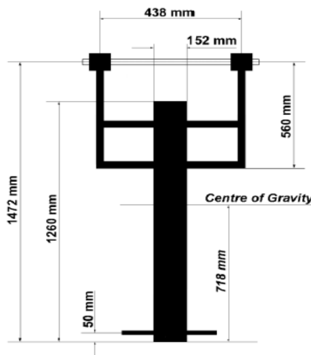
FIG. 6 PENDULUM DIMENSIONS
