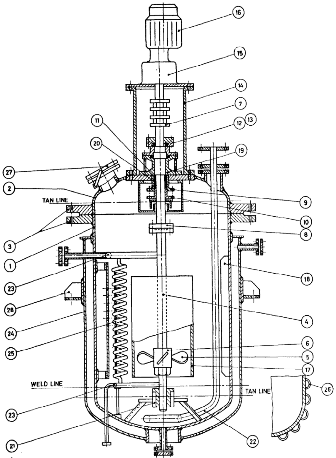
FIG. 1 AGITATOR ASSEMBLY
