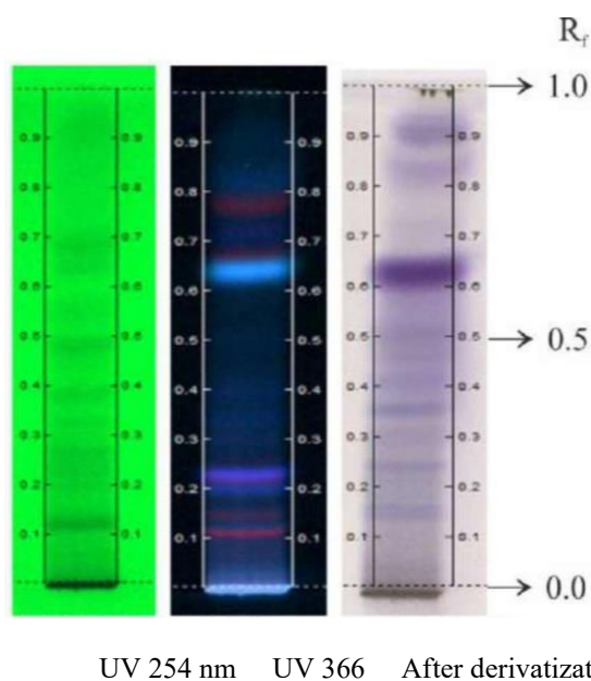
FIG. 2 TLC FINGER PRINTS OF ŪD-I BALSĀN ( COMBIPHORA OPOBALSAMUM L. ENGL.) WOOD
