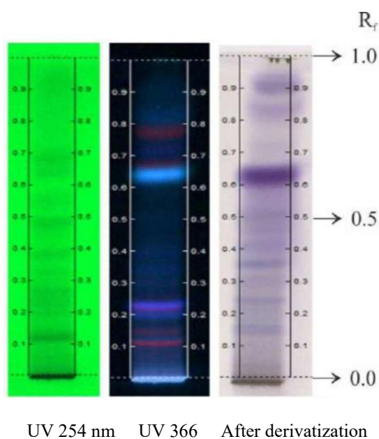
FIG.3 TLC FINGER PRINTS OF ŪD-I BALSĀN ( COMBIPHORA OPOBALSAMUM L. ENGL.) WOOD
