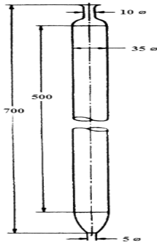
FIG. 7 PIPETTE
