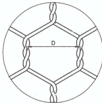
FIG. 13 MESH TYPE AND NOMINAL MESH SIZE (D)
