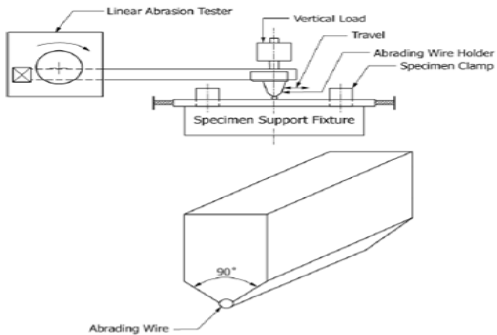
FIG. 14 LINEAR ABRADER
