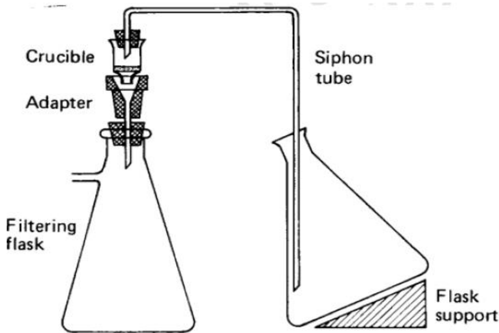
FIG. 1 LIGNIN FILTRATION APPARATUS
