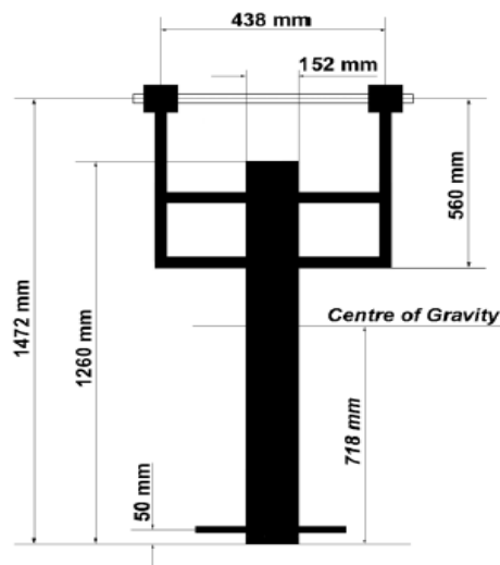
FIG. 6 PENDULUM DIMENSIONS
