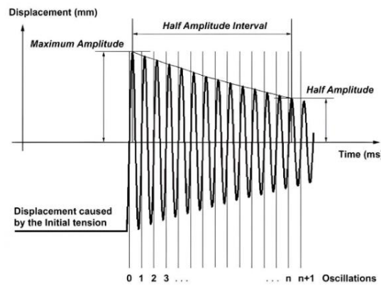
FIG. 2 OSCILLATION DAMPING PARAMETERS
