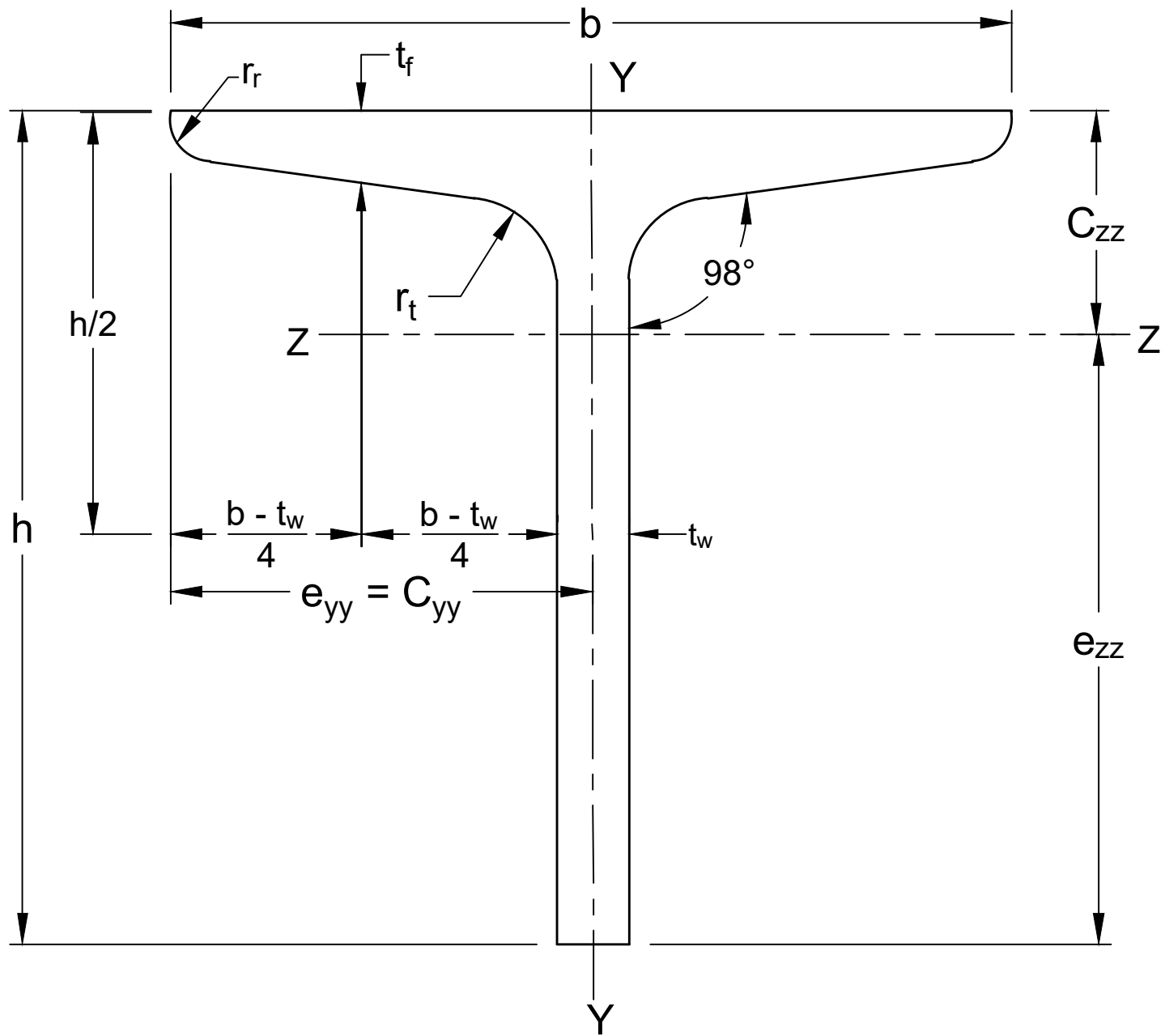
FIG. 2 SLIT TEE AND DEEP LEGGED TEE BAR
