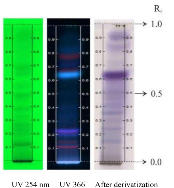
FIG.3 TLC FINGER PRINTS OF ŪD-I BALSĀN ( COMBIPHORA OPOBALSAMUM L. ENGL.) WOOD
