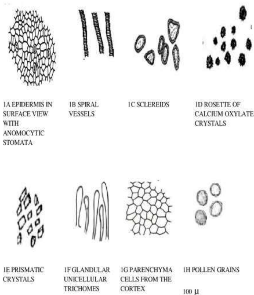
FIG. 1 GULNĀR FĀRSĪ — POWDER MICROSCOPY
